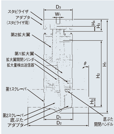
■ 拡底バケット寸法図
