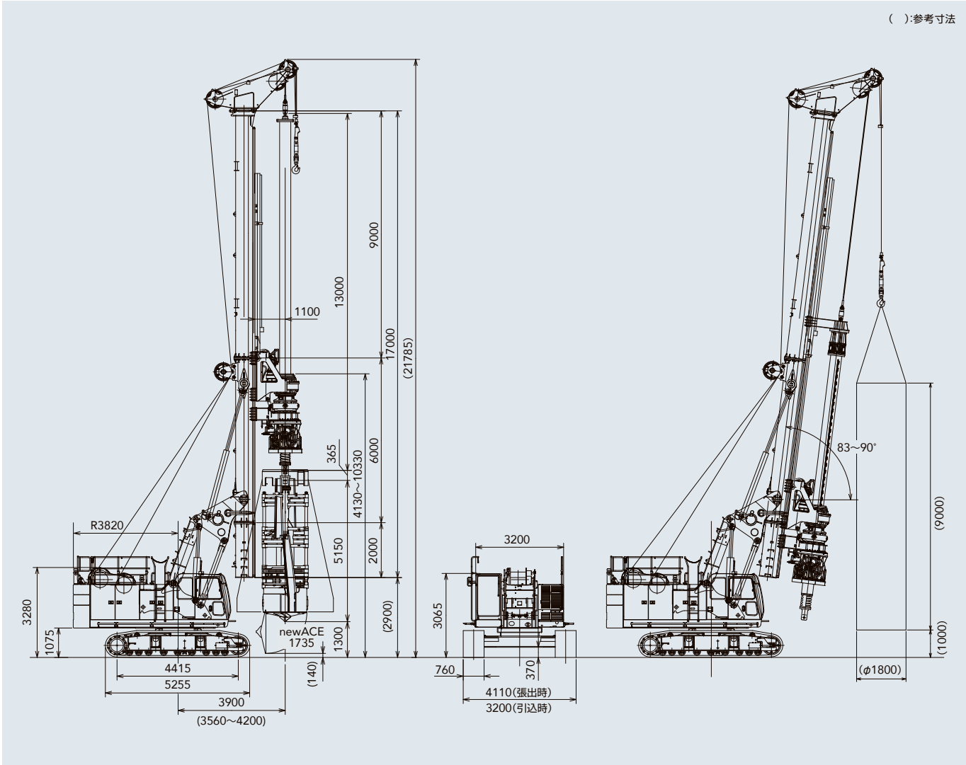
■ 寸法図
