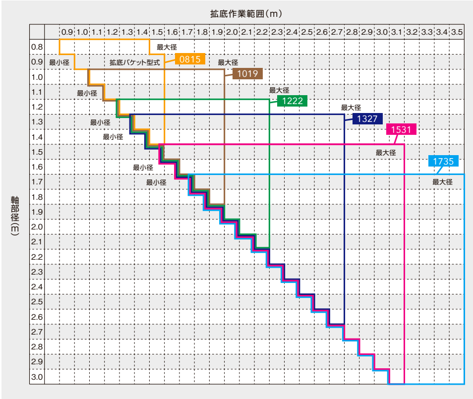
■ 拡底バケット作業範囲図 (new ACE工法)
