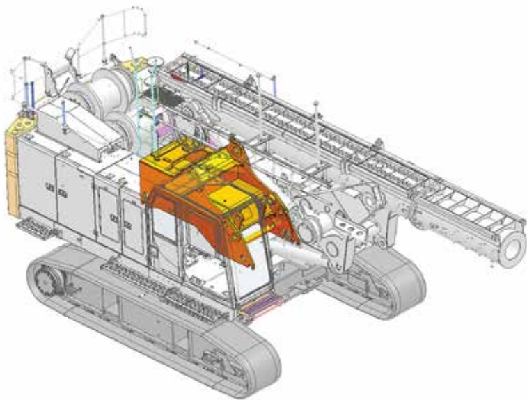
油圧シリンダ(写真はブーム式) ※写真は説明のためカバーを取り外しています。
