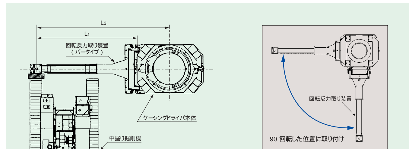
特許第2806922号(回転式ケーシングドライバの回転反力取り方法)
