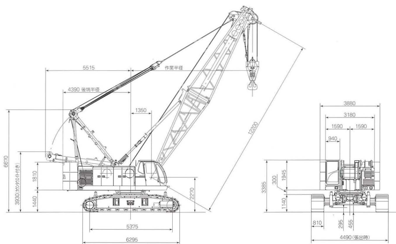
■SCX900HD-1 寸法図 (単位: mm)
