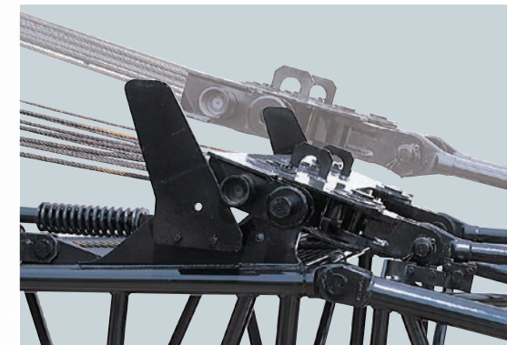
ブライドル連結ガイド ブライドルと下ブームを連結しやすくするための ガイドです。
